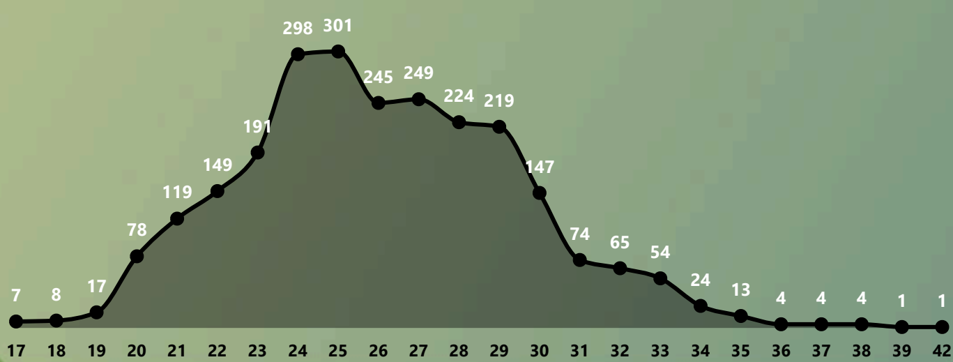
Soma de Gols por Idade
